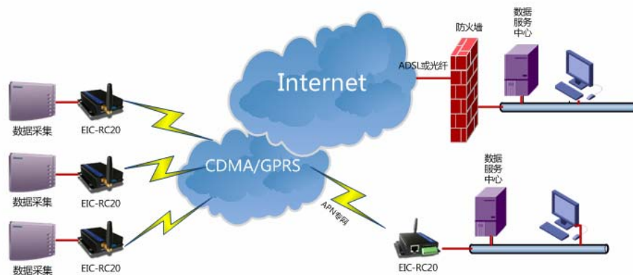
(图一) 路由远程监控系统
